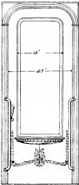
Fig. 1789. DOOR FOR PULLMAN EXTENDED VESTIBULE.
